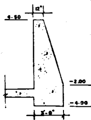
SECTION D. D
